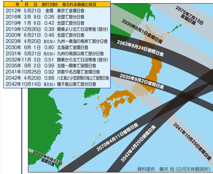
▲これから日本付近で見られる金環日食と皆既日食。表は部分日食も示しました。
