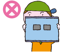
▲「日食専用グラス」の脇や上から、誤って太陽を直接見ないように注意！
