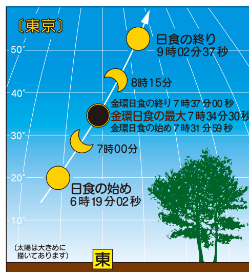
【図2 東京での見え方】 全国ほぼ同じような見え方になります。
