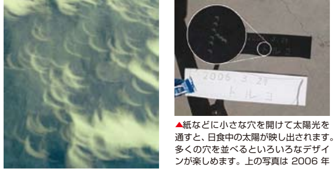
▲木の葉の間からもれた光が、たくさんの日食像となって地面に映るようすを観察することができます。
