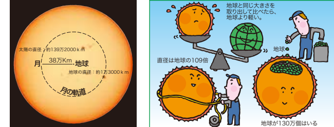
▲太陽の大きさをくらべると…… ●太陽と地球をくらべると……
